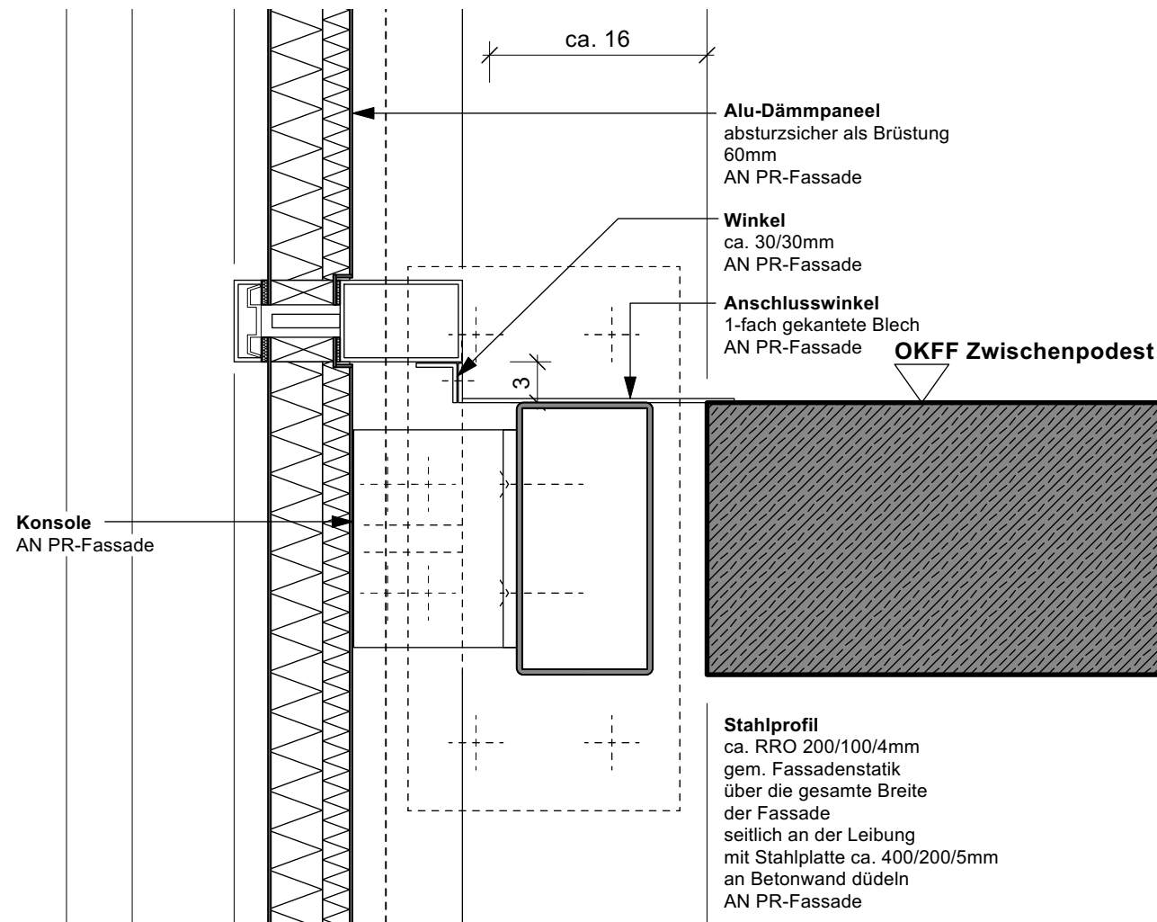
Detail 318-2 Vertikalschnitt Anschluss Zwischenpodest
