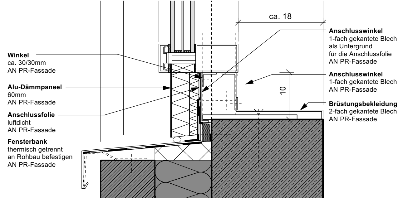
Detail 318-3 Vertikalschnitt Brüstungs- / Sockelanschluss
