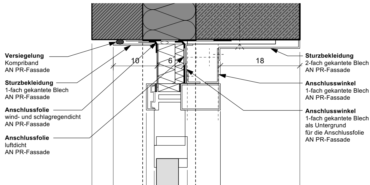
Detail 318-1 Vertikalschnitt Sturzanschluss
